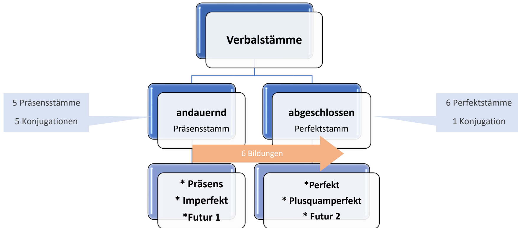
Diagramm 2: Verbalstämme 1
